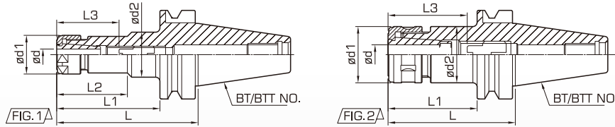
Dimensions / 尺寸標示
